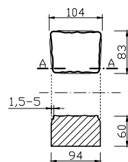
PRZEKRÓJ A-A
