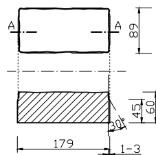
PRZEKRÓJ A-A
